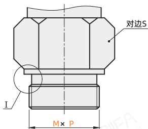
安装尺寸图
