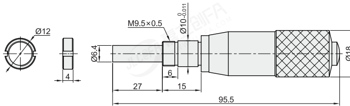
BYF62 行程：0~25(带安装螺母)
