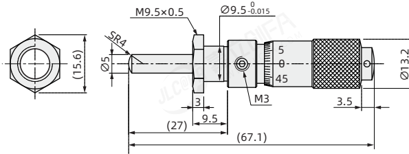
BYF26 行程：0~13(带安装螺母)
