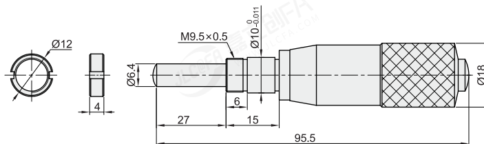
BYF72 行程：0~25(带安装螺母)
