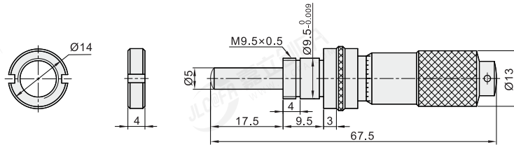
BYF24 行程：0~13(带安装螺母)
