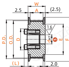
带轮形状 E形
