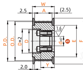
带轮形状 F形
