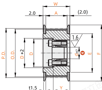
带轮形状 F形
