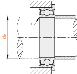
安装图
