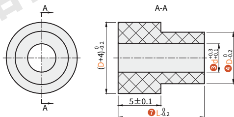
外径选择 AYHF-B/X/G-WX
