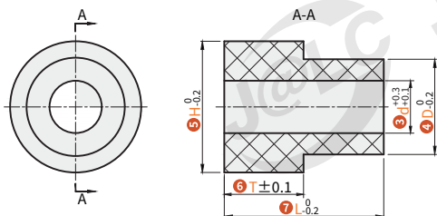
尺寸指定 AYHF-B/X/G-CD
