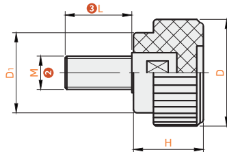
外螺纹安装 DBSN-W1
