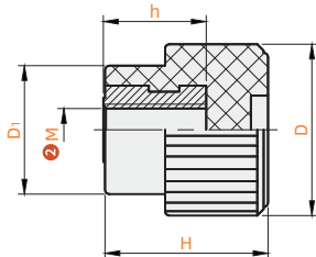
内螺纹安装 DBSN-N1
