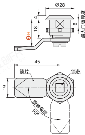
四方形 DMSY-W-4 DMSY-G3-4
