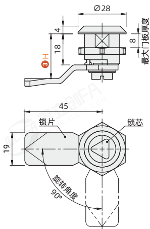
三角形 DMSY-W-3 DMSY-G3-3
