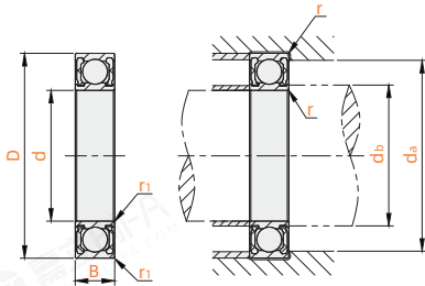
非接触式橡胶密封圈型
