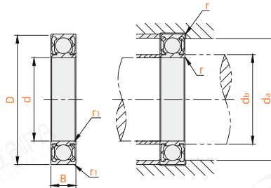
接触式橡胶密封圈型
