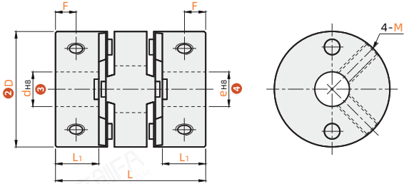
双膜片 CXGK-2
