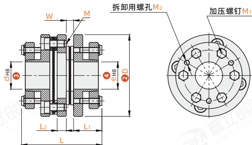
双膜片 CXGY-2
