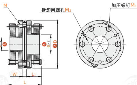
单膜片 CXGY-1
