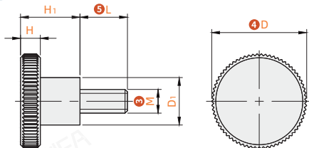
外螺纹安装 DBSQ-G2-W1
