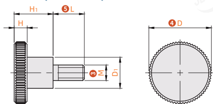
外螺纹安装 DBSQ-E1-W1/DBSQ-G3-W1/DBSQ-X3-W1
