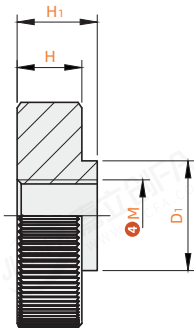
内螺纹安装 DBSU-C8G3-N1 DBSU-S3X3-N1
