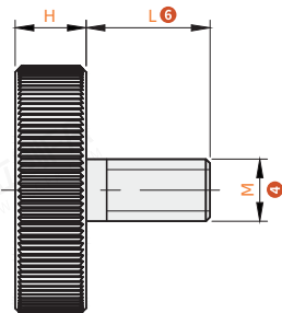
外螺纹安装 DBSU-C5G3-W1 DBSU-S3X3-W1
